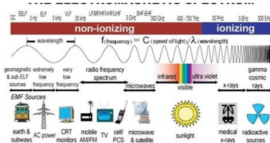
Figure 16 EM Spectrum
